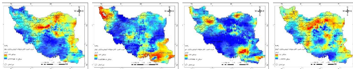
شکل ۱۵. نقشه ضریب تعیین تابش موج بلند خروجی گذر روز و بارش آوریل، می، ژوئن و فصل بهار (۲۰۱۹-۲۰۰۳)
