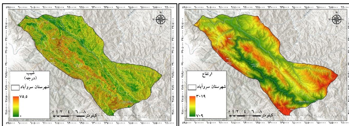
شکل ۳. نقشه شیب منطقه مورد مطالعه
