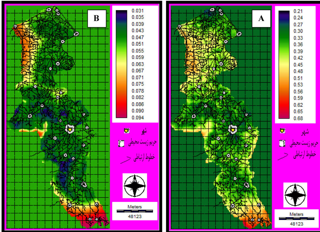
تصویر شماره ۸: A: شاخص مطلوبیت B: شاخص ناراضیاتی، تلفیق زیرمعیارها
