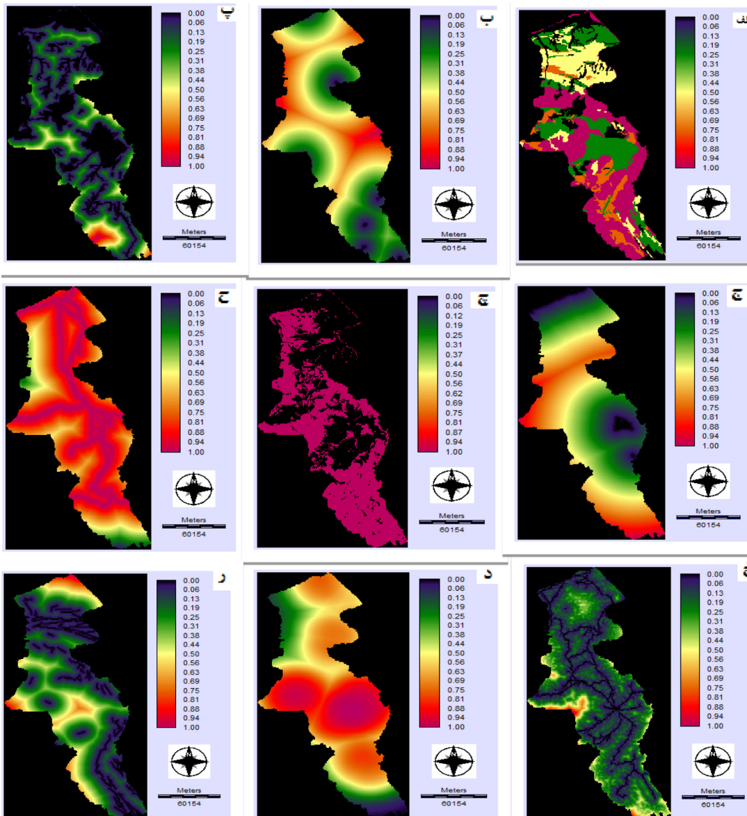
تصویر شماره ۶: استانداردسازی معیارها، (الف) زمین‌شناسی، (ب): فاصله از دریاچه‌ها، (پ): فاصله از آبخوان، (ج): فاصله از دشت‌های سیلابی، (چ) فاصله از زمین‌های کشاورزی، (ح): فاصله از خطوط انتقال برق، (خ) فاصله از راه‌های ارتباطی، (د): فاصله از وزنه‌های جمعیتی و (ر): فاصله از خطوط گسل.
